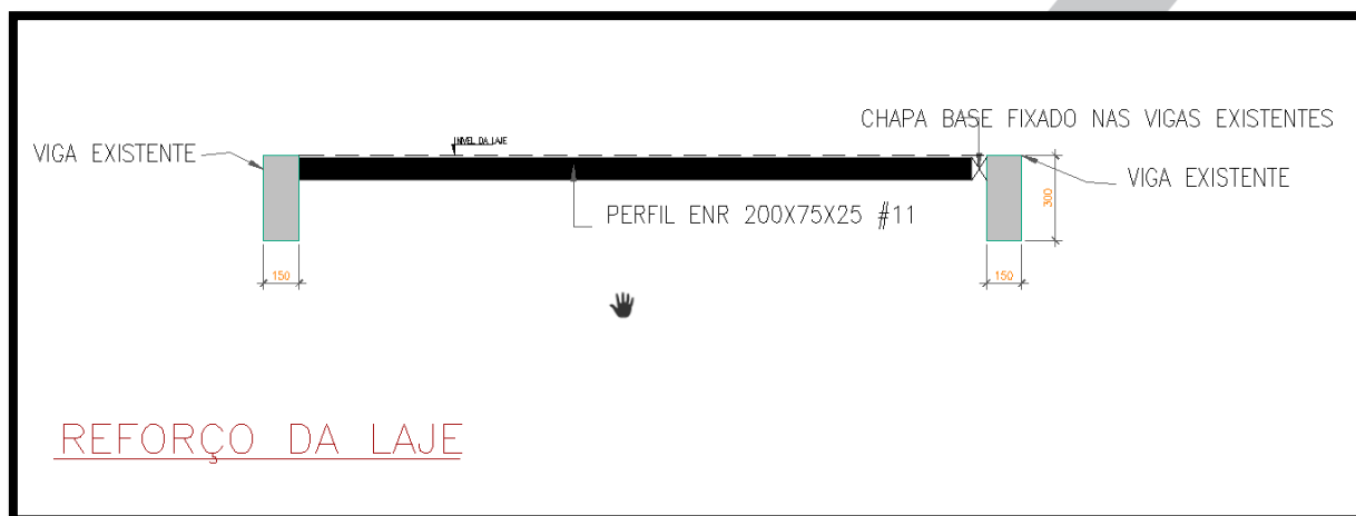
Figura 5- REFORÇO SUPORTE DA LAJE
