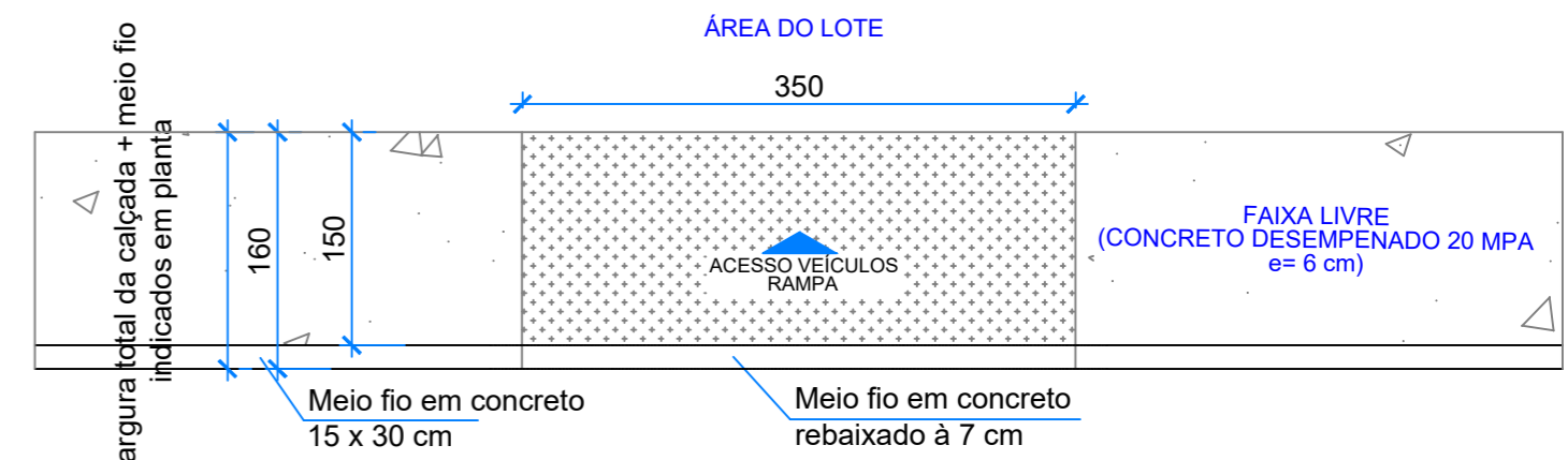
Detalhe de rebaixo para acesso de veículos
