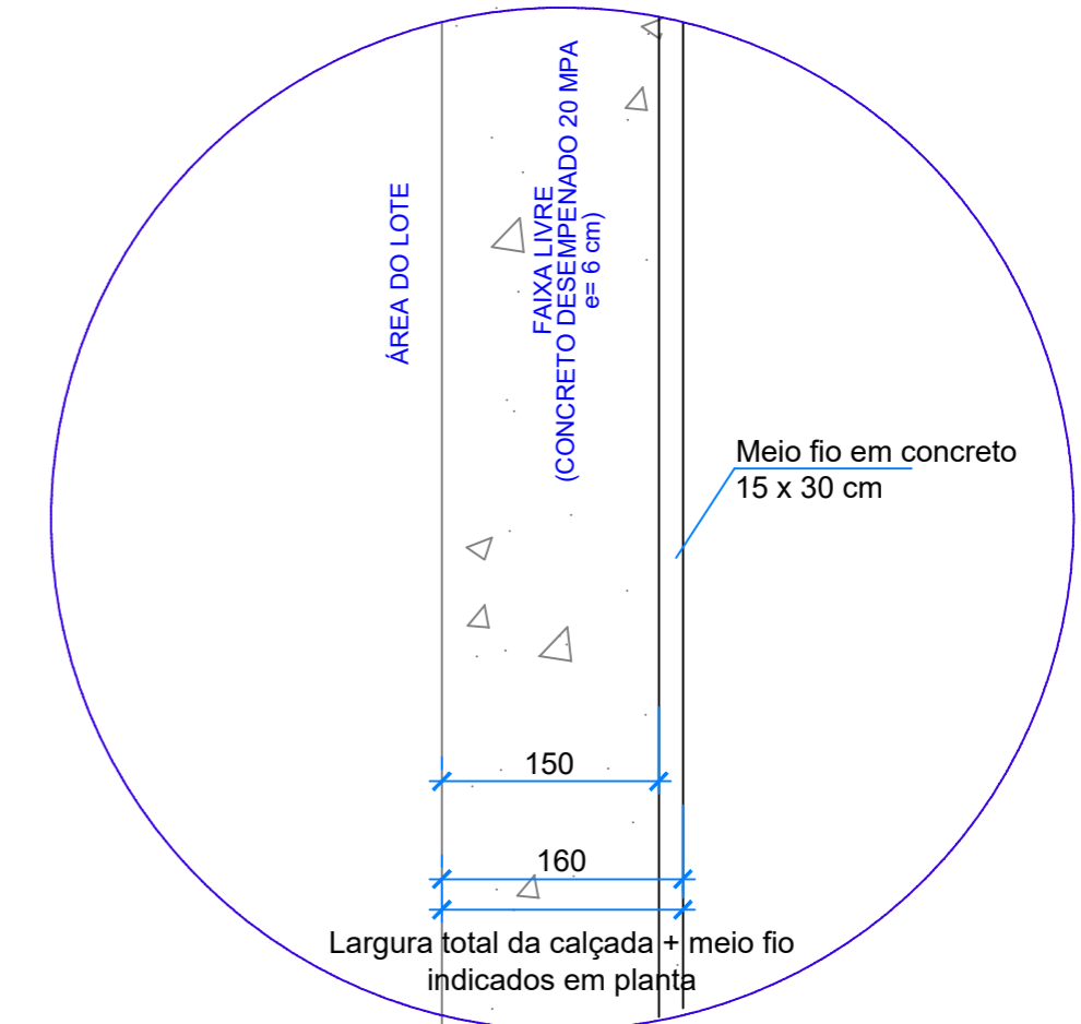
Detalhe geral de calçada
