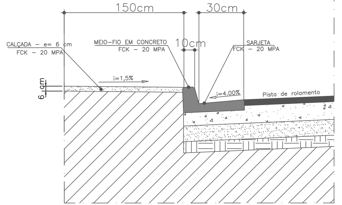
SEÇÃO TRANSVERSAL DA CALÇADA Largura de 1,50 m
