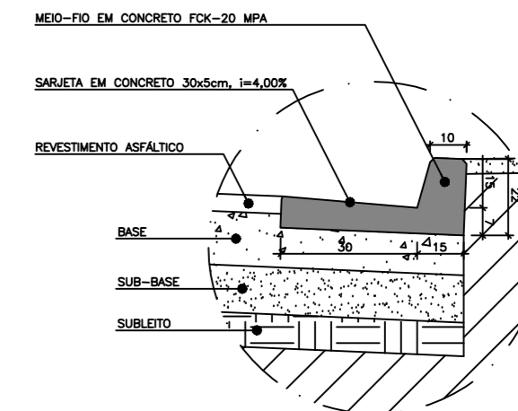
DETALHE 02 – MEIO-FIO E SARJETA
