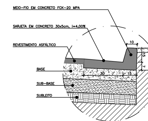
DETALHE 01 – MEIO-FIO E SARJETA
