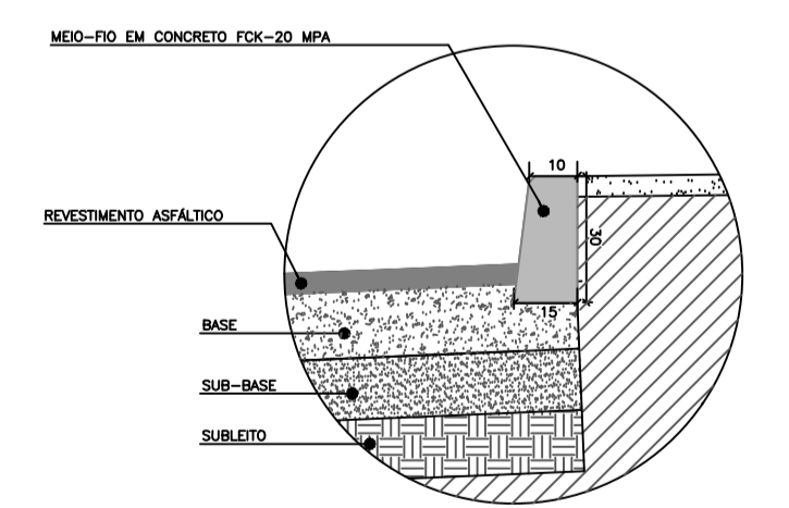
DETALHE 02 – MEIO-FIO
