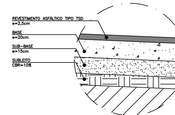
DETALHE 01 – CORTE CAMADAS TSD TRÁFEGO MÉDIO
