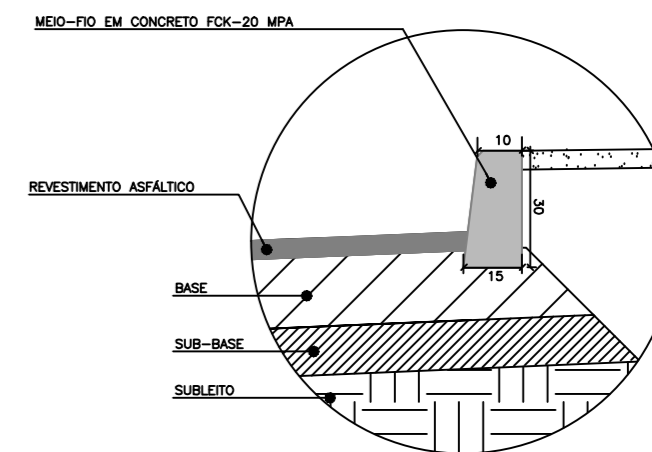
DETALHE 03 – MEIO-FIO
