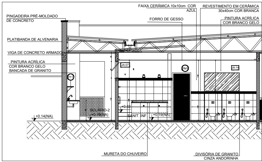
CORTE - SANIT. INFANTIL ESC/1: 25
