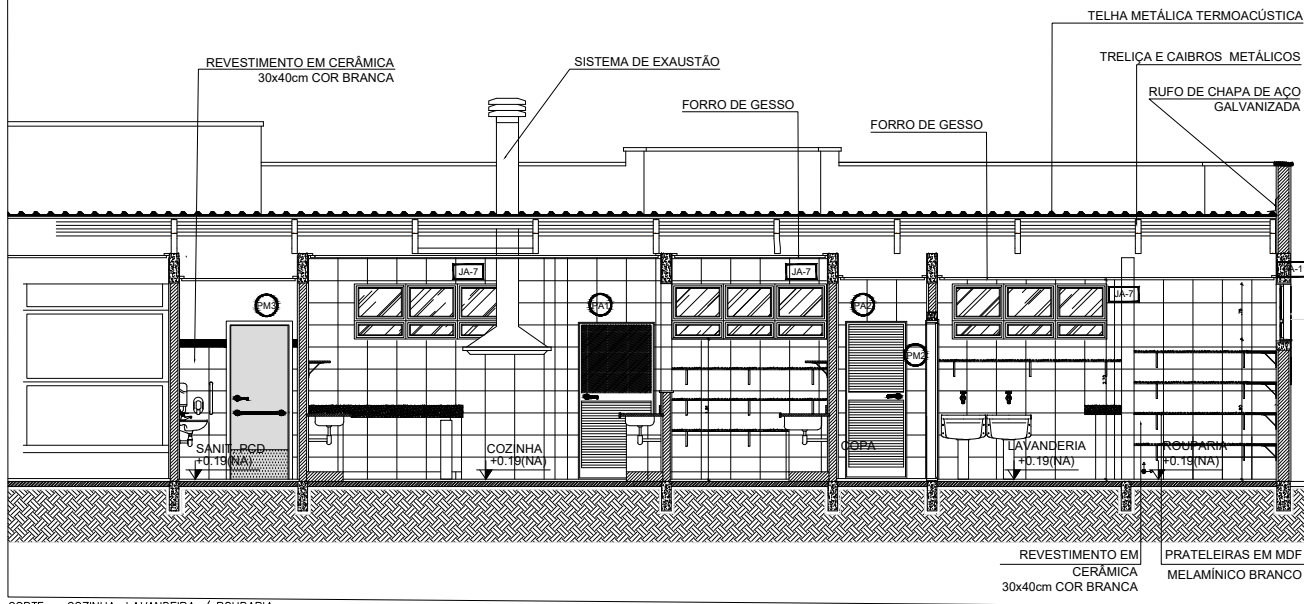
CORTE - COZINHA, LAVANDEIRA / ROUPARIA ESC/1: 25
