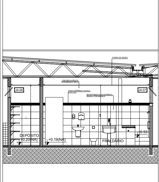
CORTE - FRALDÁRIO ESC/1: 25
