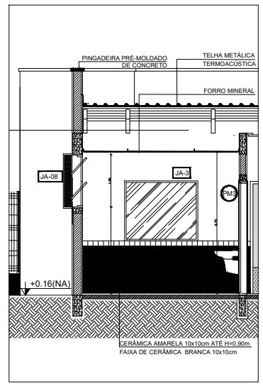
CORTE - AMAMENTAÇÃO ESC/1: 25
