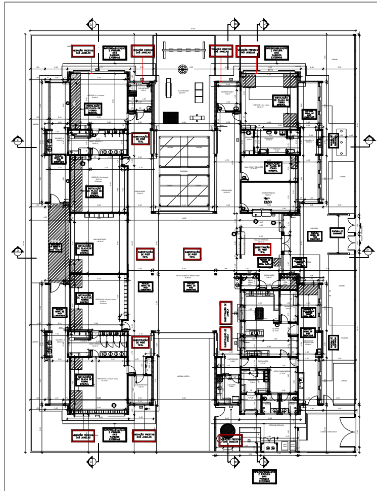
Planta Baixa 1:100
