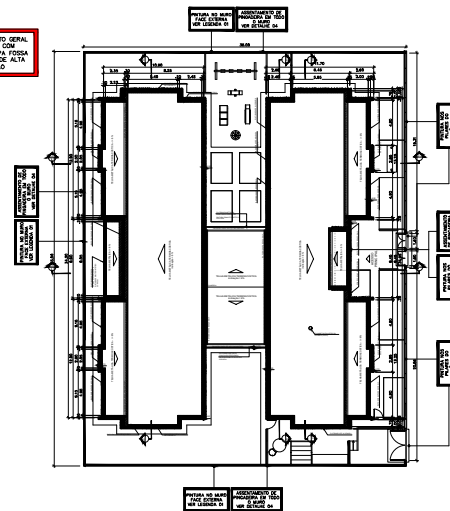
Planta de Cobertura 1:200
