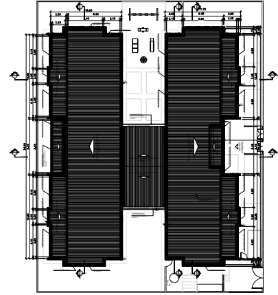
Planta de Cobertura 1:200
