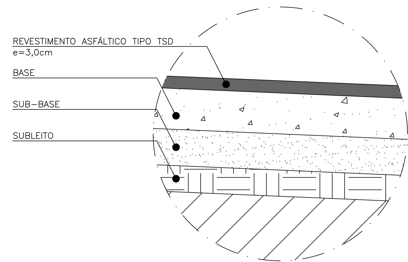
DETALHE 01
