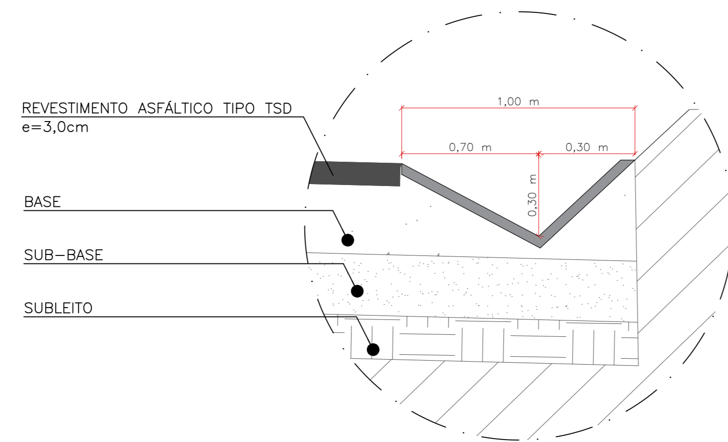
DETALHE 02
