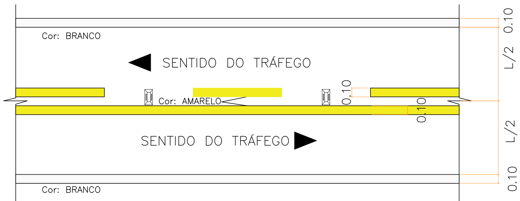
DETALHE SINALIZAÇÃO HORIZONTAL Esc:1/25
