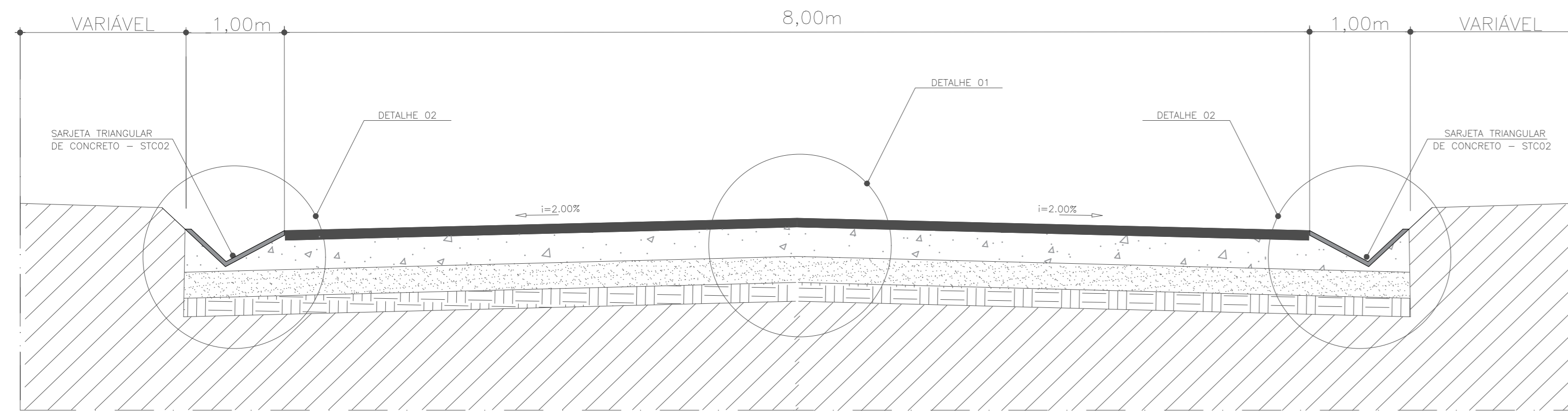
CORTE TRANSVERSAL PISTA DE ROLAMENTO - PAV. ASFÁLTICO Largura de 8,00 m
