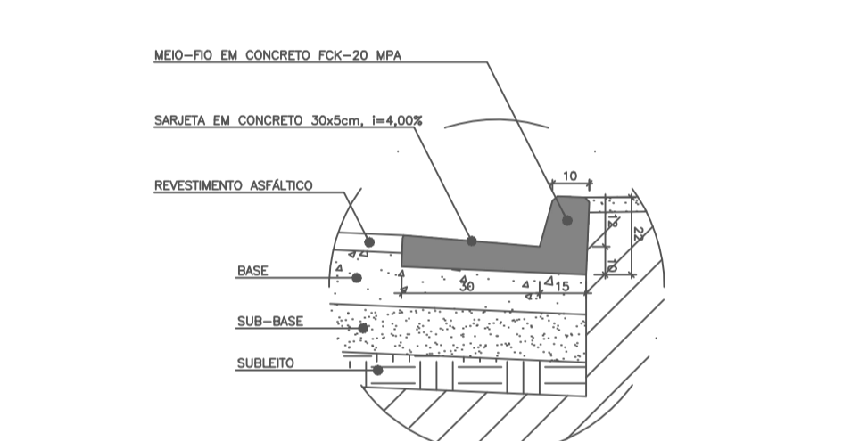
DETALHE 02 - MEIO-FIO E SARJETA - PAV. ASFÁLTICO
