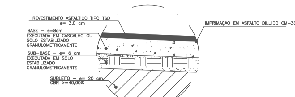
DETALHE 01 - CORTE CAMADAS Tráfego Muito Leve
